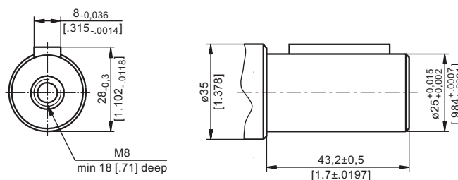
CA - \phi 25 straight, Parallel key A8x7x32 DIN 6885 Max. Torque 34 daNm [3010 lb-in]
