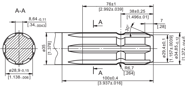
SL - \phi 34,85 p.t.o. DIN 9611 Form 1 Max. Torque 77 daNm [6815 lb-in]
